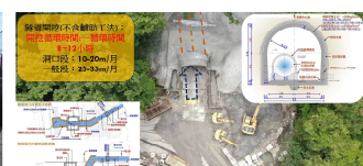
NATM施工現場（俯瞰）
