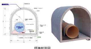
標準断面図
