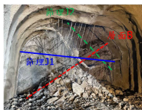
施工中の変状（施工時の状況写真）
